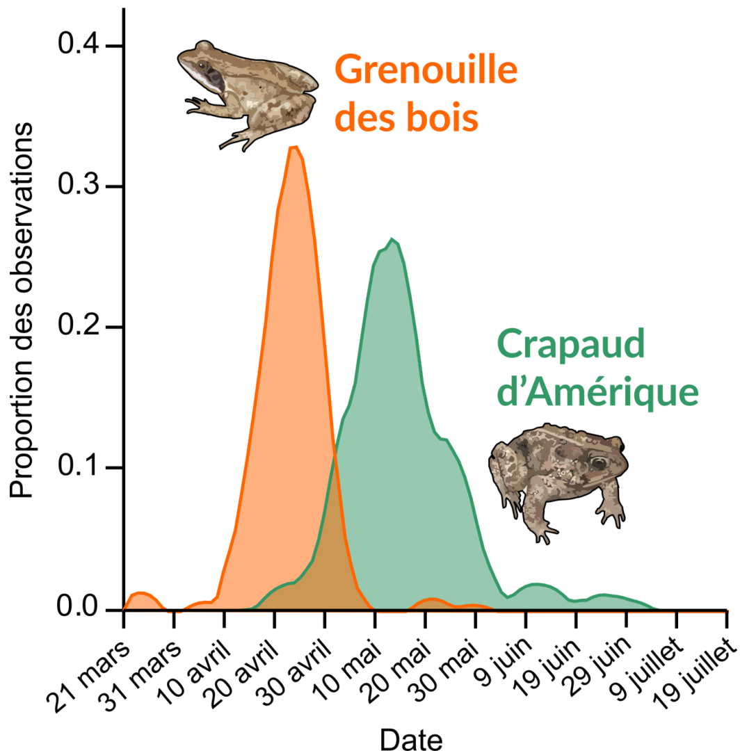
Figure 1. Fréquence d'observation des choroales (cote 3) pour la grenouille des bois et le crapaud d'Amérique en fonction de la date dans la zone climatique A (5.0 à 6.5°C) de 1993 à 2018. Notez bien la période de reproduction plus courte de la grenouille des bois comparativement à celle du crapaud. Bien que les deux espèces peuvent être entendues en même temps, notez également l'écart entre les pics de choroales des deux espèces.
